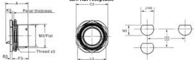
Jam nut receptacle
