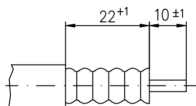
Kabelzuschnitt
